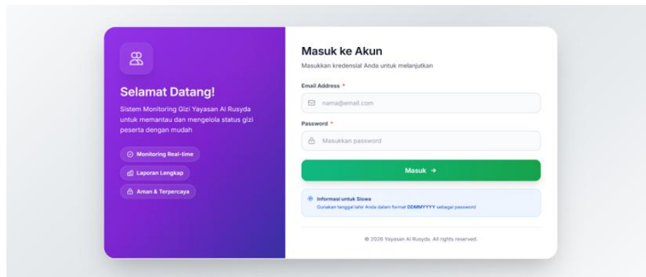
Gambar 4. Halaman Login
