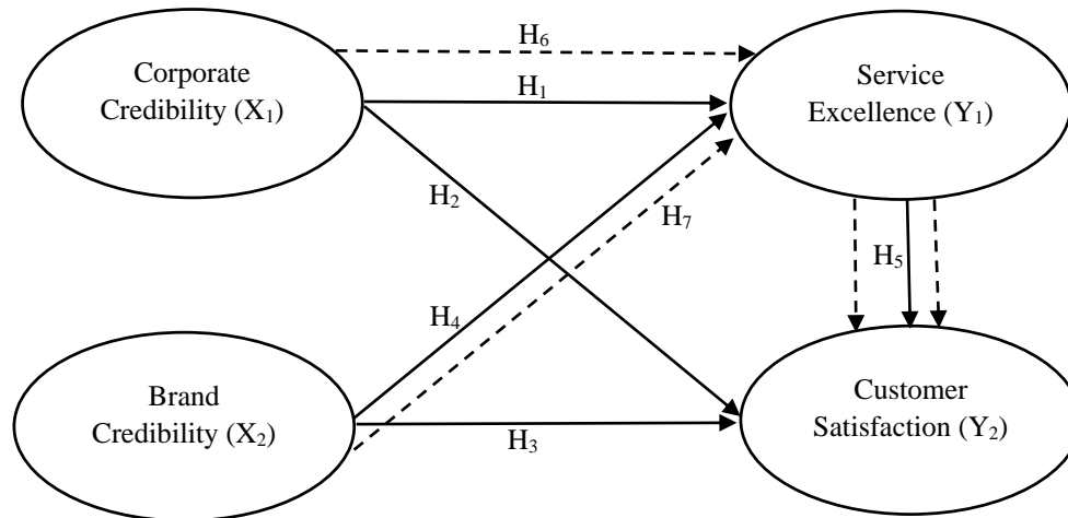
Gambar 1. Kerangka Berpikir
