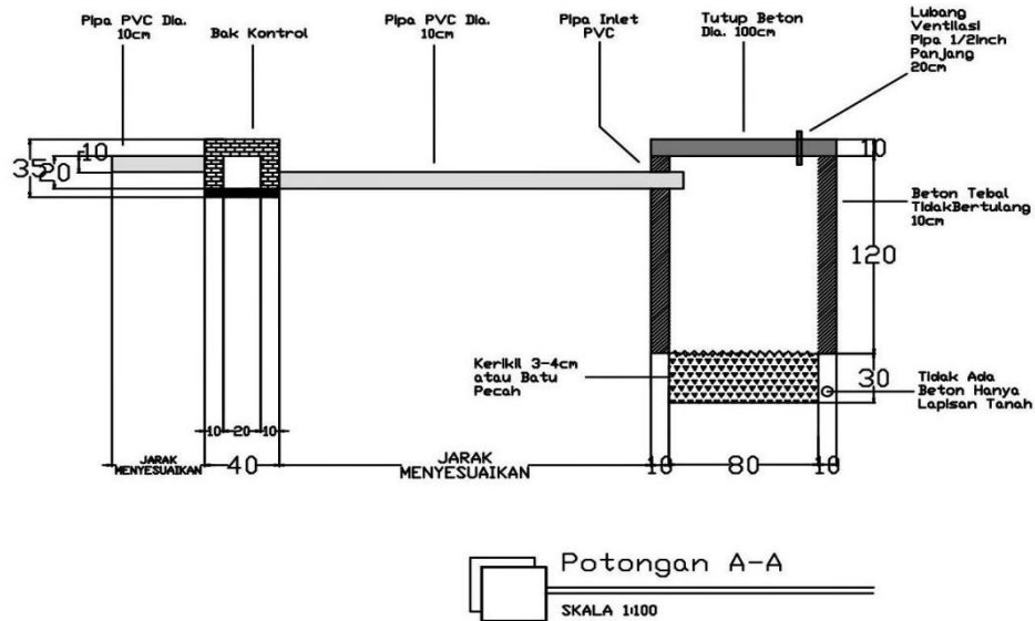
Gambar 6. Potongan A - A Sarana Saluran Pembuangan Air Limbah (SPAL)
