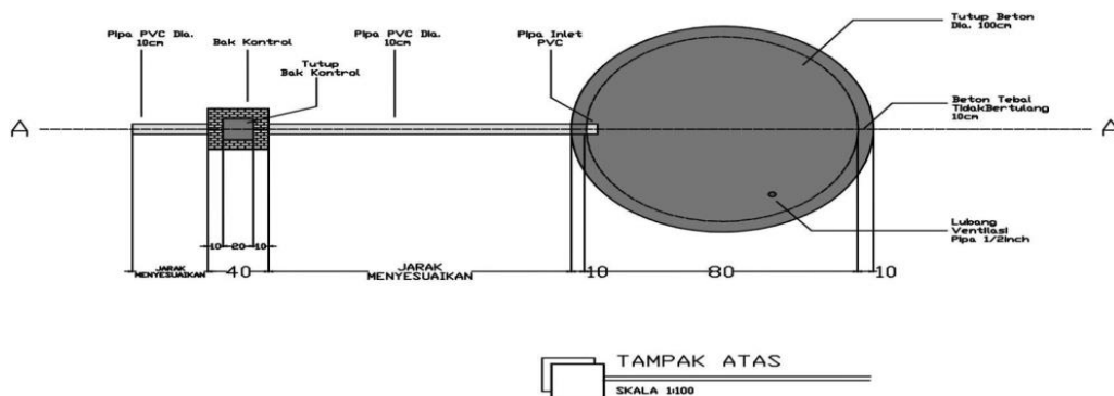
Gambar 5. Denah Tampak Atas Pembuangan Air Limbah (SPAL)
