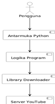
Gambar 2. Arsitektur Sistem
