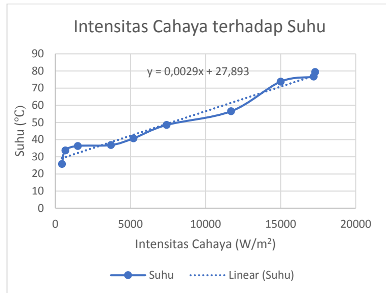
Gambar 8. Grafik Intensitas Cahaya terhadap suhu
