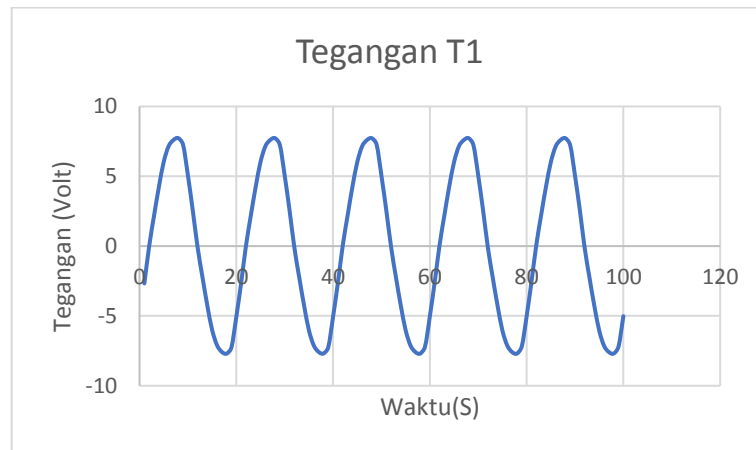
Gambar 4. Tegangan T1 sebelum di kalibrasi dengan acuan 200V
