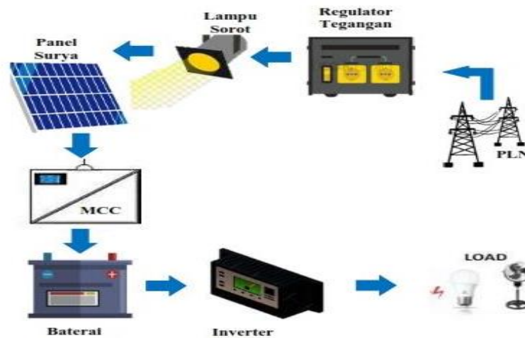
Gambar 1. Desain Penelitian
