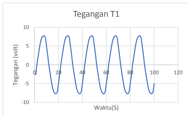
Gambar 6. Tegangan T1 sesudah di kalibrasi
