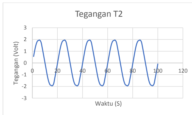
Gambar 5. Tegangan T2 sebelum di kalibrasi dengan acuan 200V
