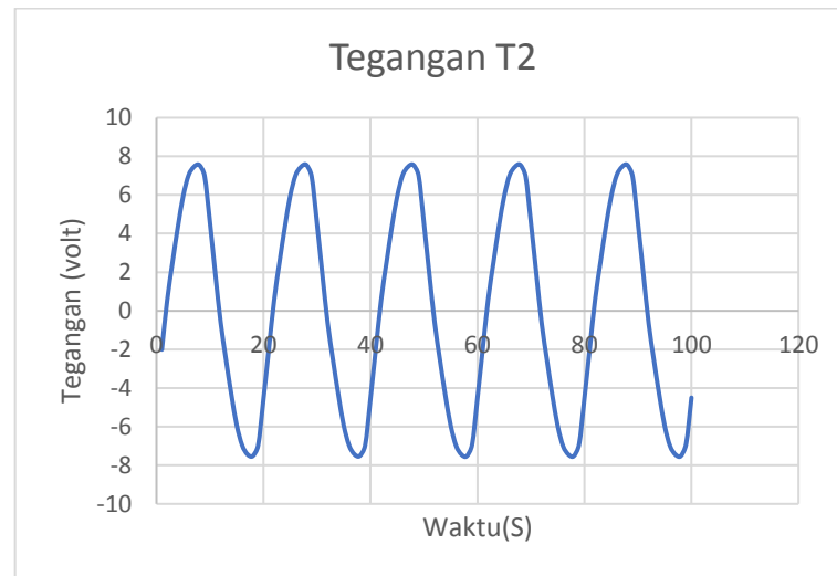
Gambar 7. Tegangan T2 sesudah di kalibrasi
